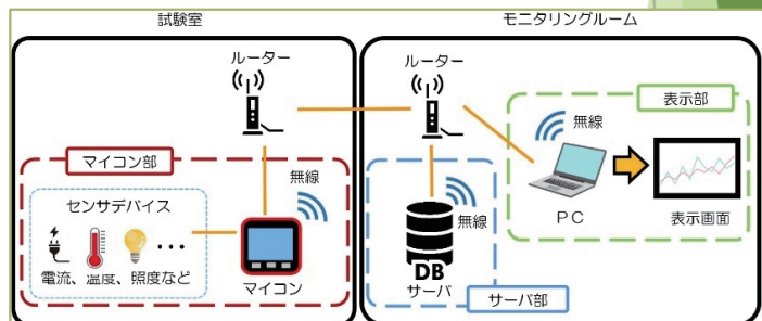
例2) 工作機械の稼働状況の可視化
