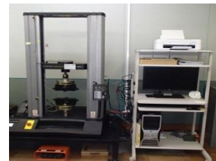
万能引張試験機(5kN) インストロン 5565
